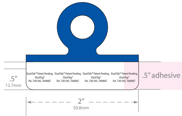
Die #2243
