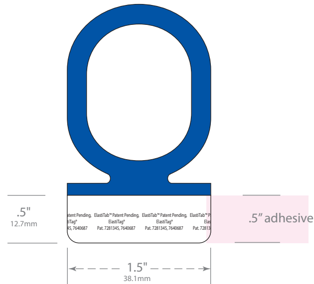
Die #2164
