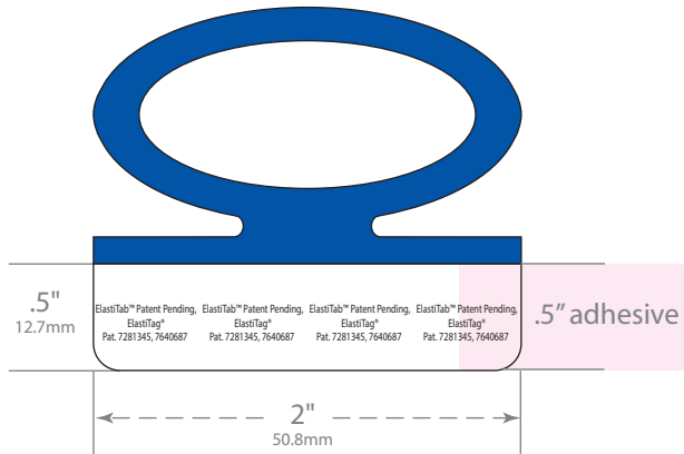
Die #2102
