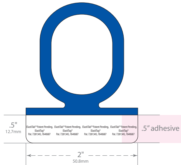
Die #2145
